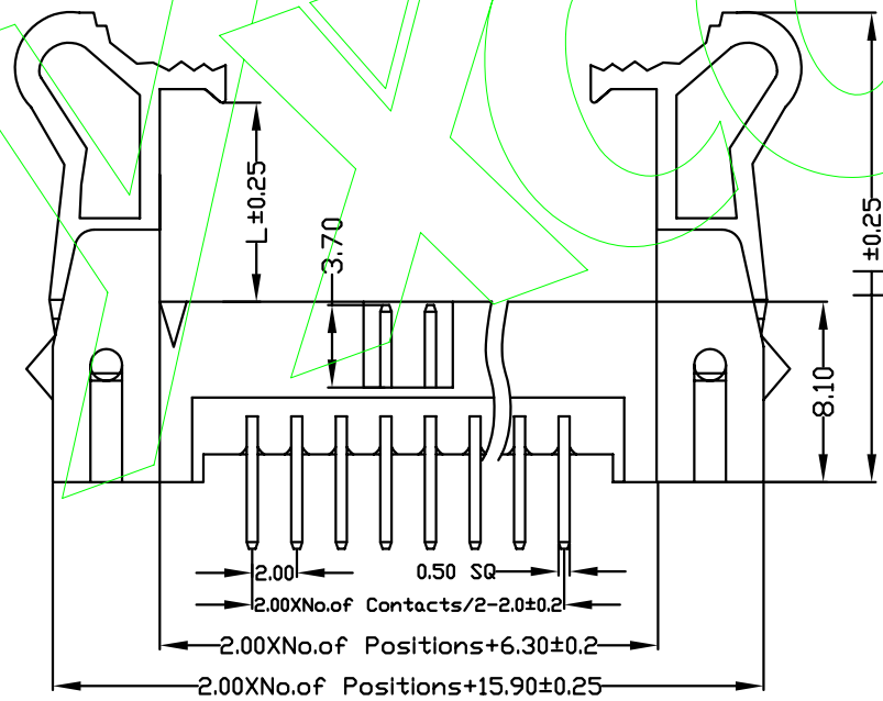
Long Latch
